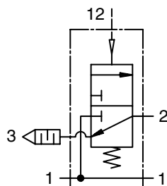
SB.01 I pneum. Betätigung
